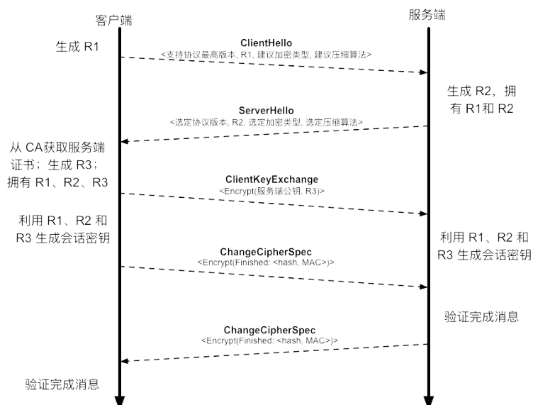
图 1.8.3.2 - TLS 握手协商过程
