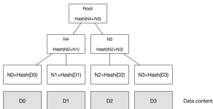
图 1.8.7.1 - Merkle 树示例
