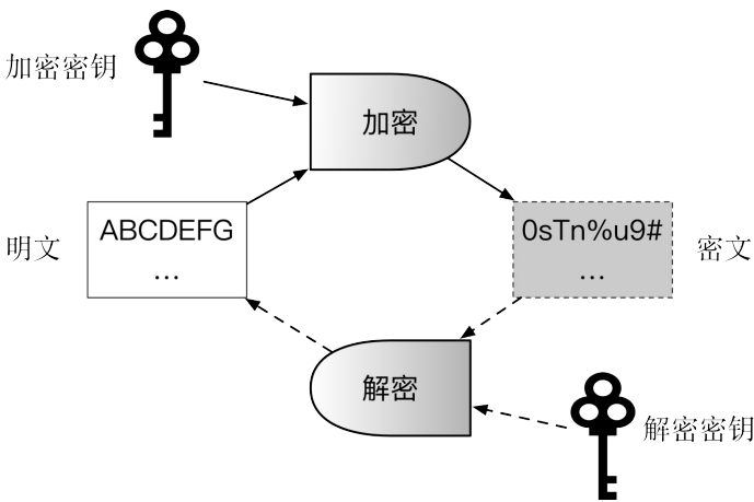
图 1.8.3.1 - 加解密的基本过程
