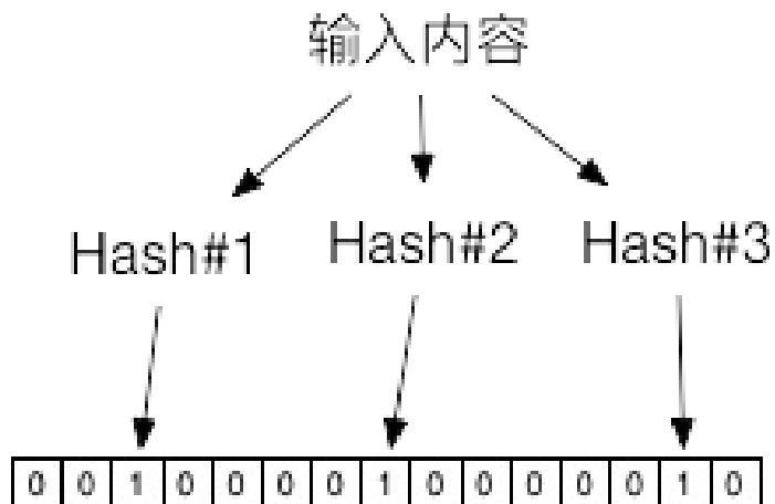
图 1.8.8.1 - 布隆过滤器
